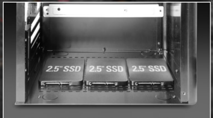
機殼底部 硬碟/SSD 不同配置安裝方式
